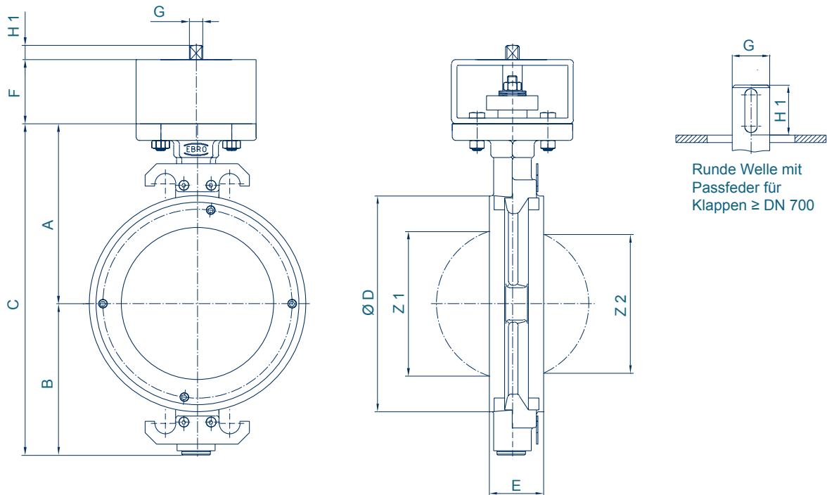
HP 111 mit freiem Wellenende gem. EN ISO 5211
